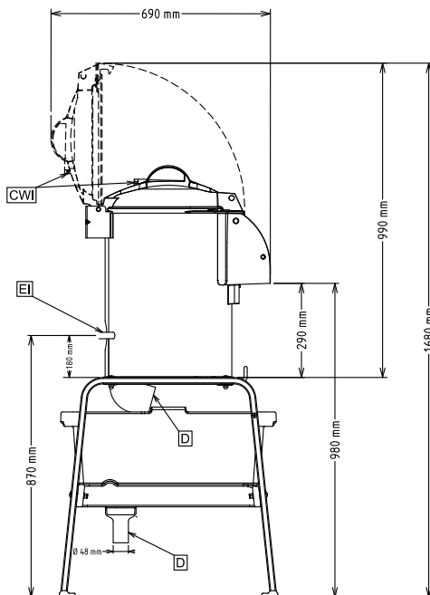
Zij aanzicht
